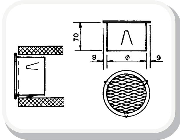
Ventilationseinsätze aus Stahlblech, feuerverzinkt
